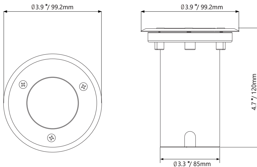
LT2206A
