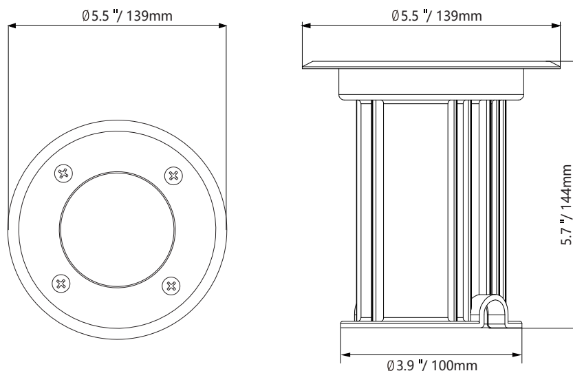
LT2206B
